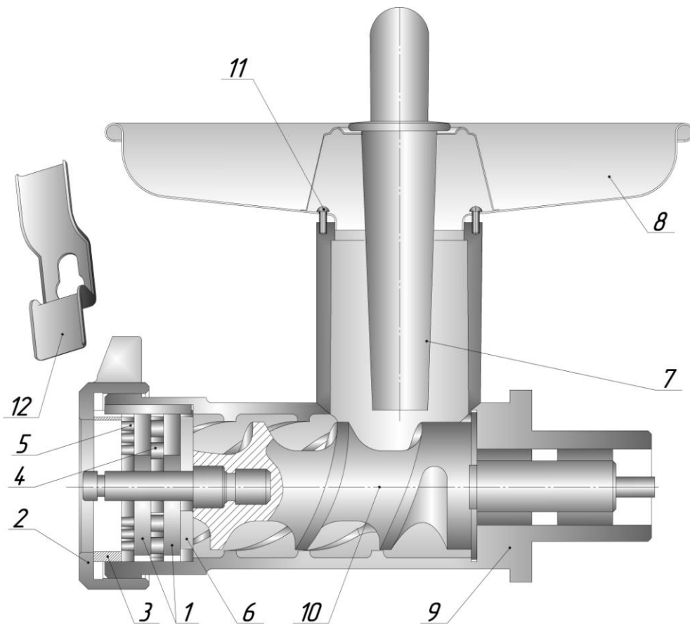
Рисунок 2 – Мясорубка ММ
